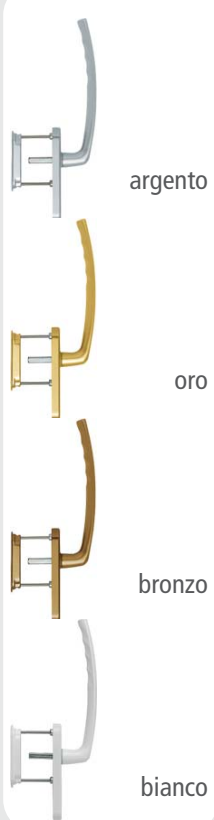
modello ATLANTA tipo maniglione singolo con maniglietta da incasso esterna versione standard materiale alluminio
